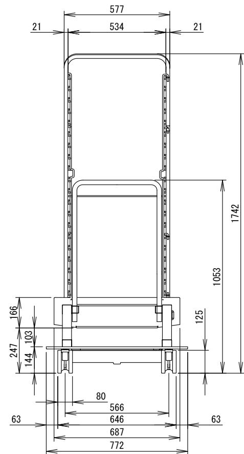
型式 20-2/1 ラックレールの間隔（ピッチ）
